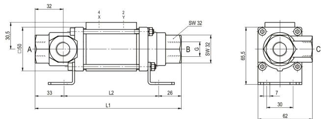
CVTE3-10 Funkció NO
