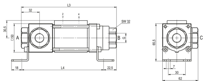
CVTE3-10 Funkció NC (> 63bar)
