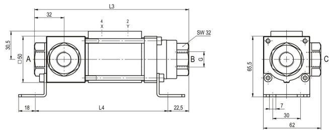
CVTE3-10 Funkció NO (> 63bar)
