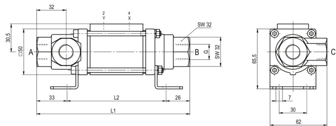
CVTE3-10 Funkció NC
