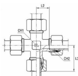
mit B4-Schneidring
