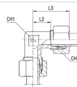
mit B3-Schneidring
