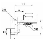
mit B4-Schneidring
