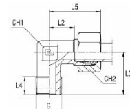
mit B3-Schneidring
