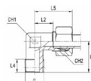
mit B3-Schneidring
