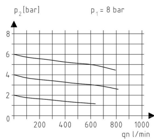
Átfolyási diagram
