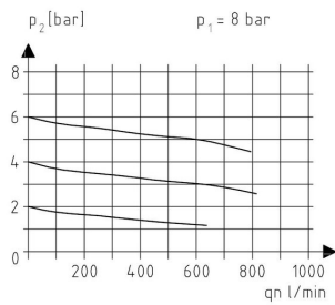
Wykres przepływu
