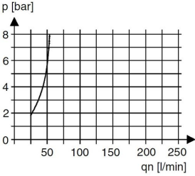
Öler-Ansprechgrenze
