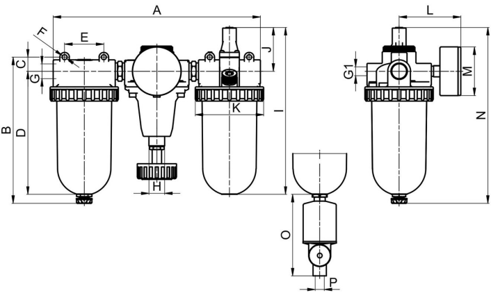
automatisches Ablassventil
