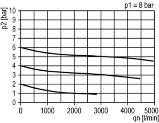
Durchflussdiagramm
