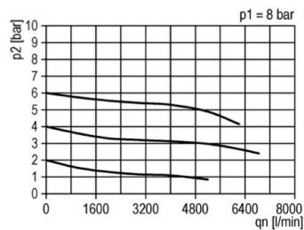
Durchflussdiagramm
