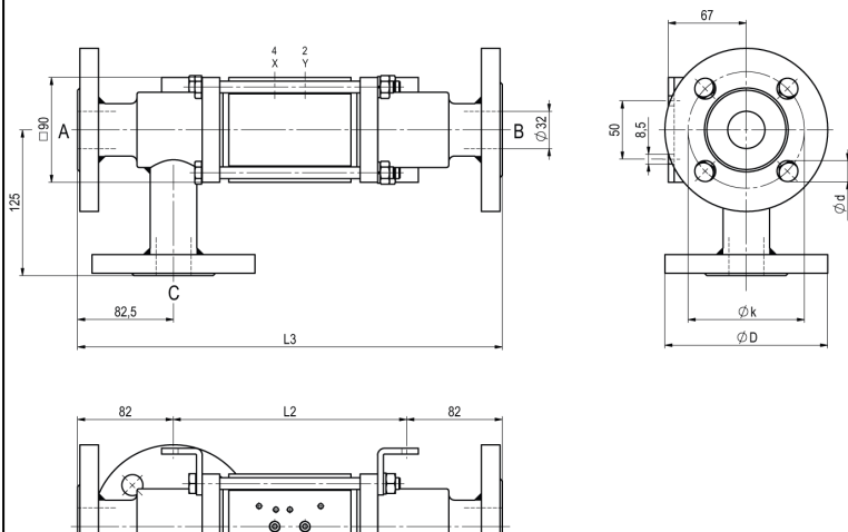
CVFE3-32 Funktion NO
