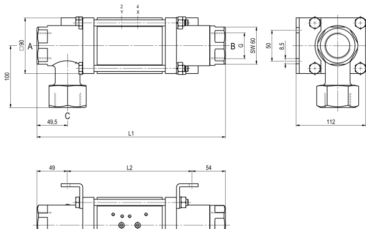
CVTE3-32 Funktion NC
