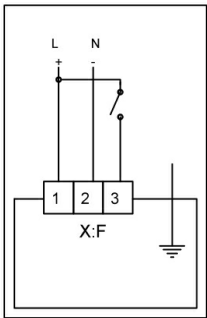
2-Punkt-Ansteuerung
