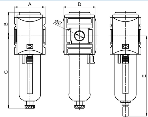
halbautomatisches Ablassventil
