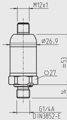
mit Rundstecker M12 x 1 (4-polig, metallisch)
