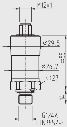
mit Rundstecker M12 x 1 ( 4-polig)
