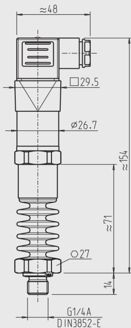
mit Winkelstecker DIN 175301-803 A und Kühlstrecke
