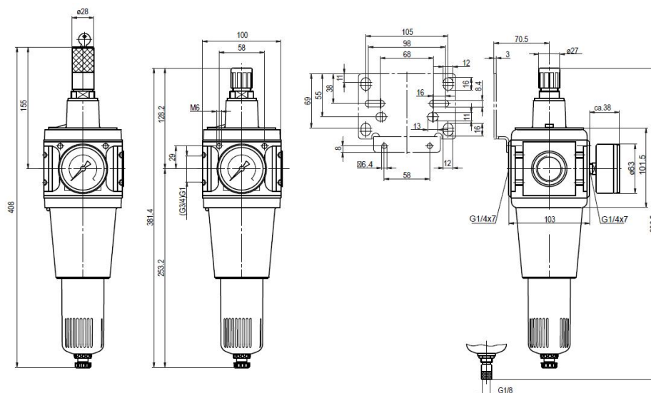
félautomata leeresztőszelep
