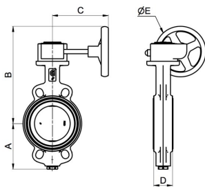
Vmesna prirobnična izvedba
