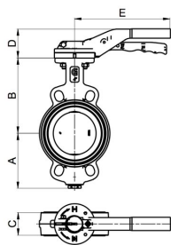
Zwischenflanschausführung
