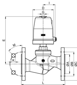
Vzmet odpre, Tip SE23
