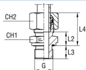
s řezným kroužkem B4
