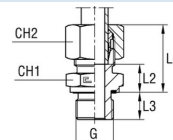
s řezným kroužkem B3
