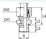
s řezným kroužkem B4
