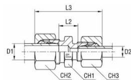
z pierścieniem zacinającym B3
