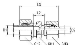
z pierścieniem tnącym B4
