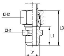
z pierścieniem tnącym B4
