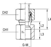
mit B4-Schneidring
