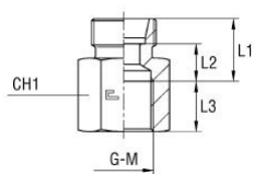
Grundkörper
