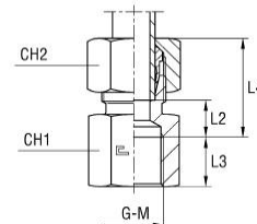
mit B3-Schneidring
