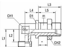
Základní těleso
