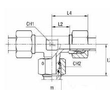
z pierścieniem zacinającym B3
