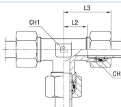
mit B4-Schneidring
