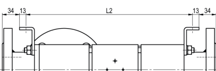
CVFV3-50 Funktion NO
