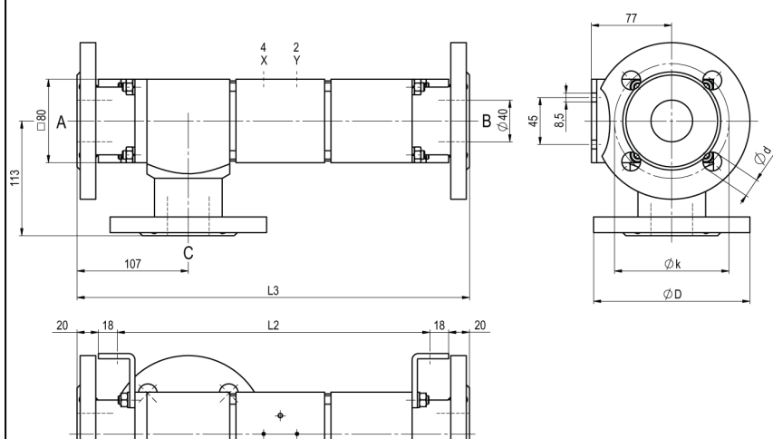
CVFV3-40 funkce NO
