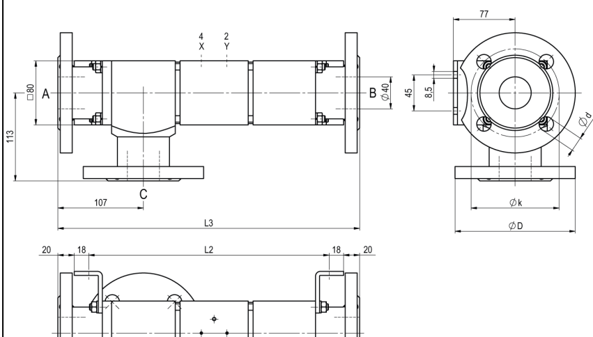
CVFV3-40 Funktion NO
