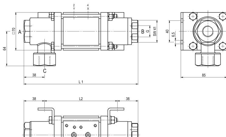
CVTE3-15 funkce NC
