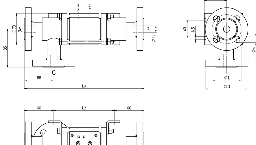
CVFE3-15 funkce NO
