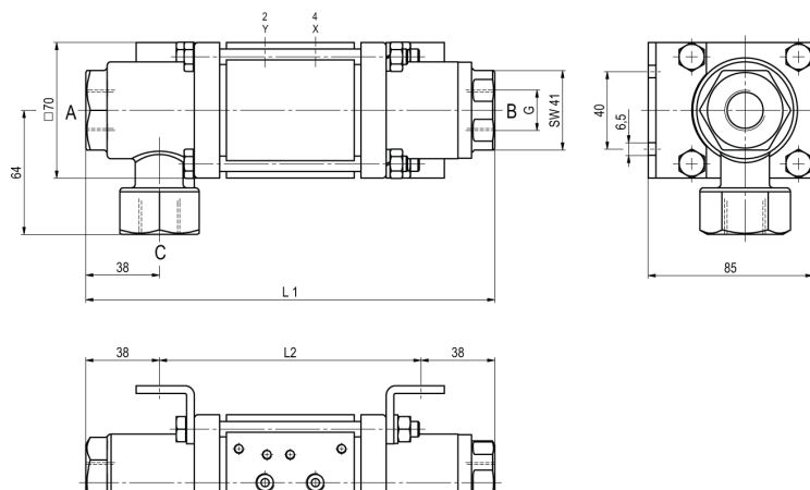
CVTE3-15 function NC
