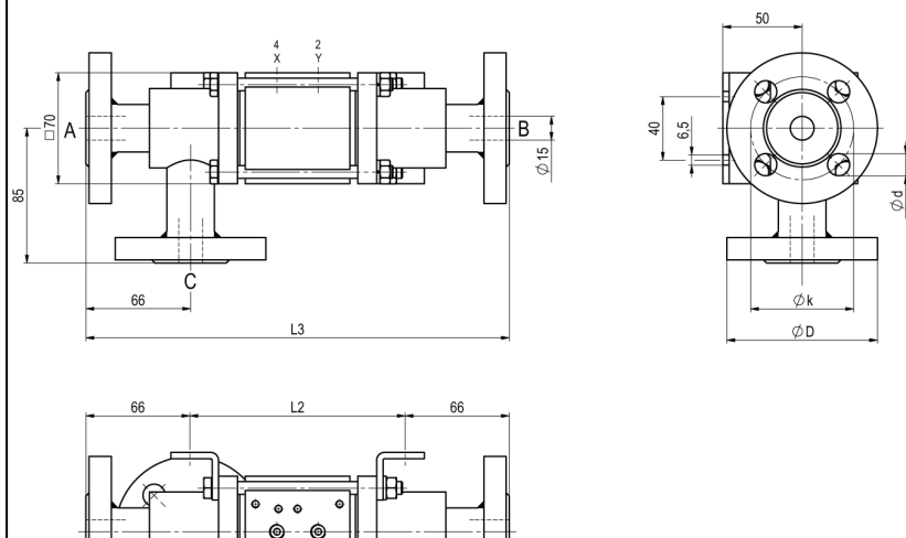
CVFE3-15 function NO
