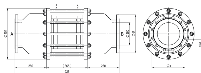
CVFV-200 funkcija NO
