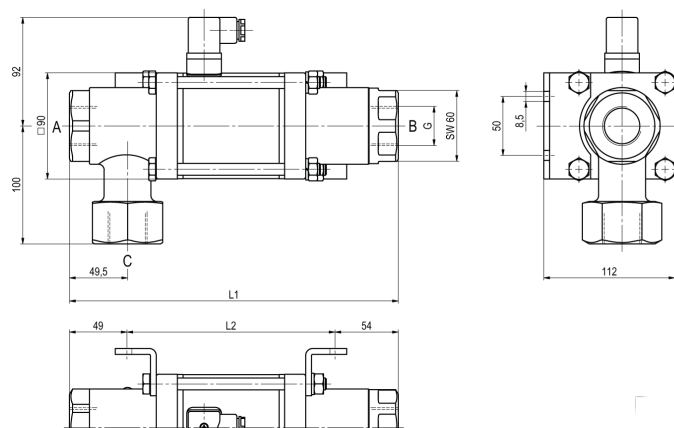
CVT3-25 funkcija NC
