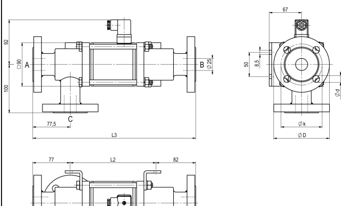
CVF3-25 funkcija NO
