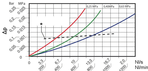
*Empfohlener maximaler Durchfluss Das Diagramm zeigt verschiedene Eingangsdrücke
