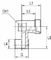
becsavarható csavarzatok
