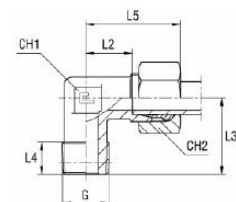
B3-as vágógyűrűvel
