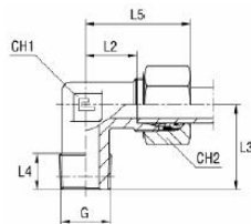
B4-es vágógyűrűvel
