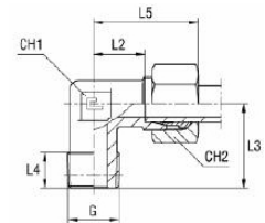
B3-as vágógyűrűvel
