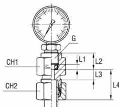
z pierścieniem tnącym B4
