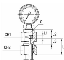
z pierścieniem zacinającym B3
