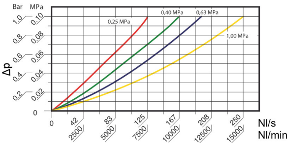
Diagram zobrazuje různé vstupní tlaky až do max. poklesu tlaku 1bar
