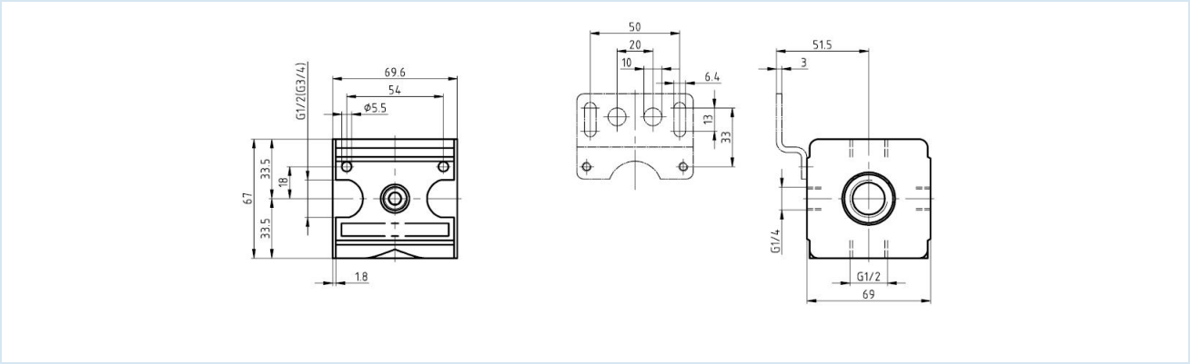
Rysunek wymiarowy do podłączenia G1/2" i G3/4"
