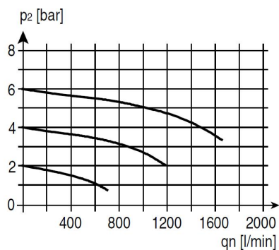
šema tehnološkog procesa
