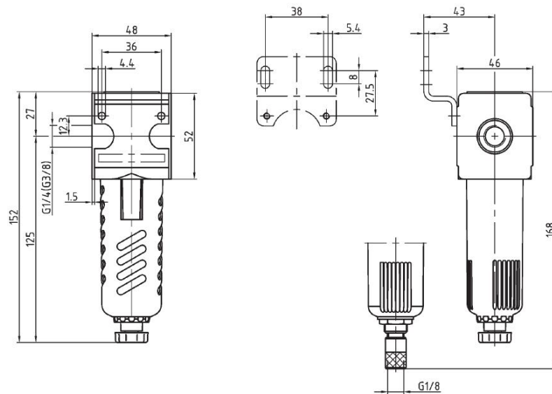
automatisches Ablassventil
