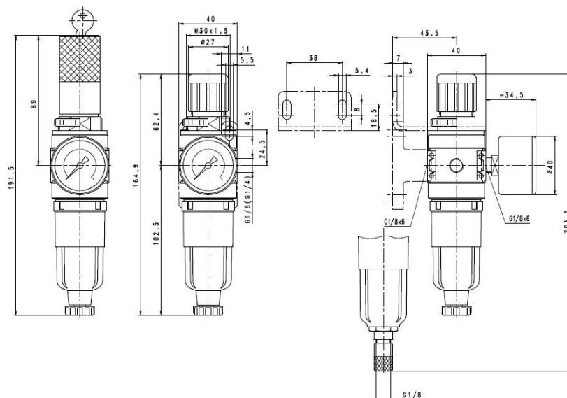
félautomata leeresztőszelep
