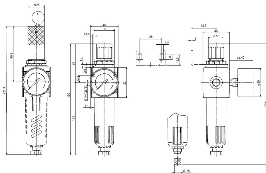
félautomata leeresztőszelő
