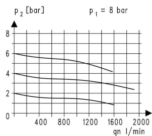
Wykres przepływu
