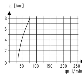
Öler-Ansprechgrenze
