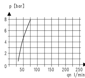
Öler-Ansprechgrenze
