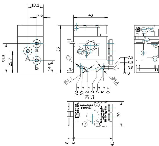
Maßzeichnung
