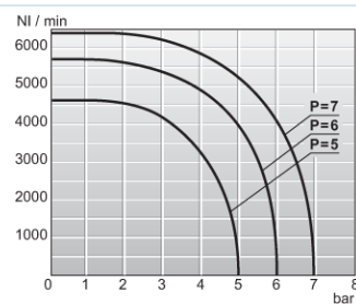
Průtokový diagramm 1/2"
